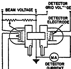
Klystron detector circuit.
